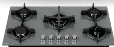
DG 527 سرشعله های SABAF راندمان بالا (HE) شیشه شات طوسی ایتالیا Size: 920x520 mm Cut: 840x475 mm
